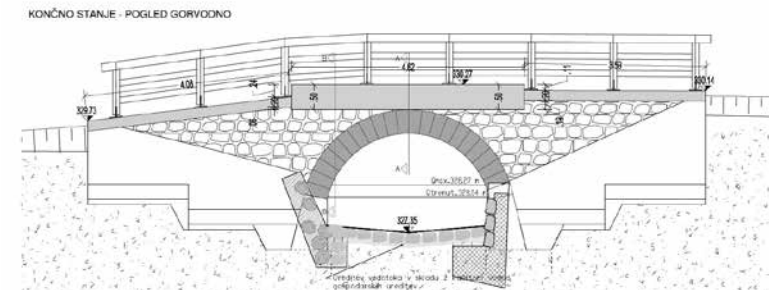
Začetni projektantski predlog PNZ, d. o. o., za sanacijo mostu (po obstoječem stanju).
