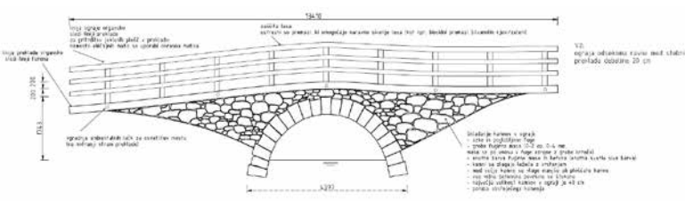
Predlog ZVKDS (avtor načrta Uroš Gantar): Organski (v obliki krivulje) potek linije ograje z debelino betonske kape 20 cm ter sonaravnim in avtentičnim zlaganjem kamnov
